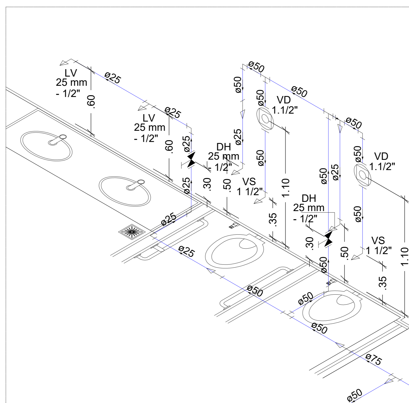
Detalhe Isometrico H2 Escala 1:25
