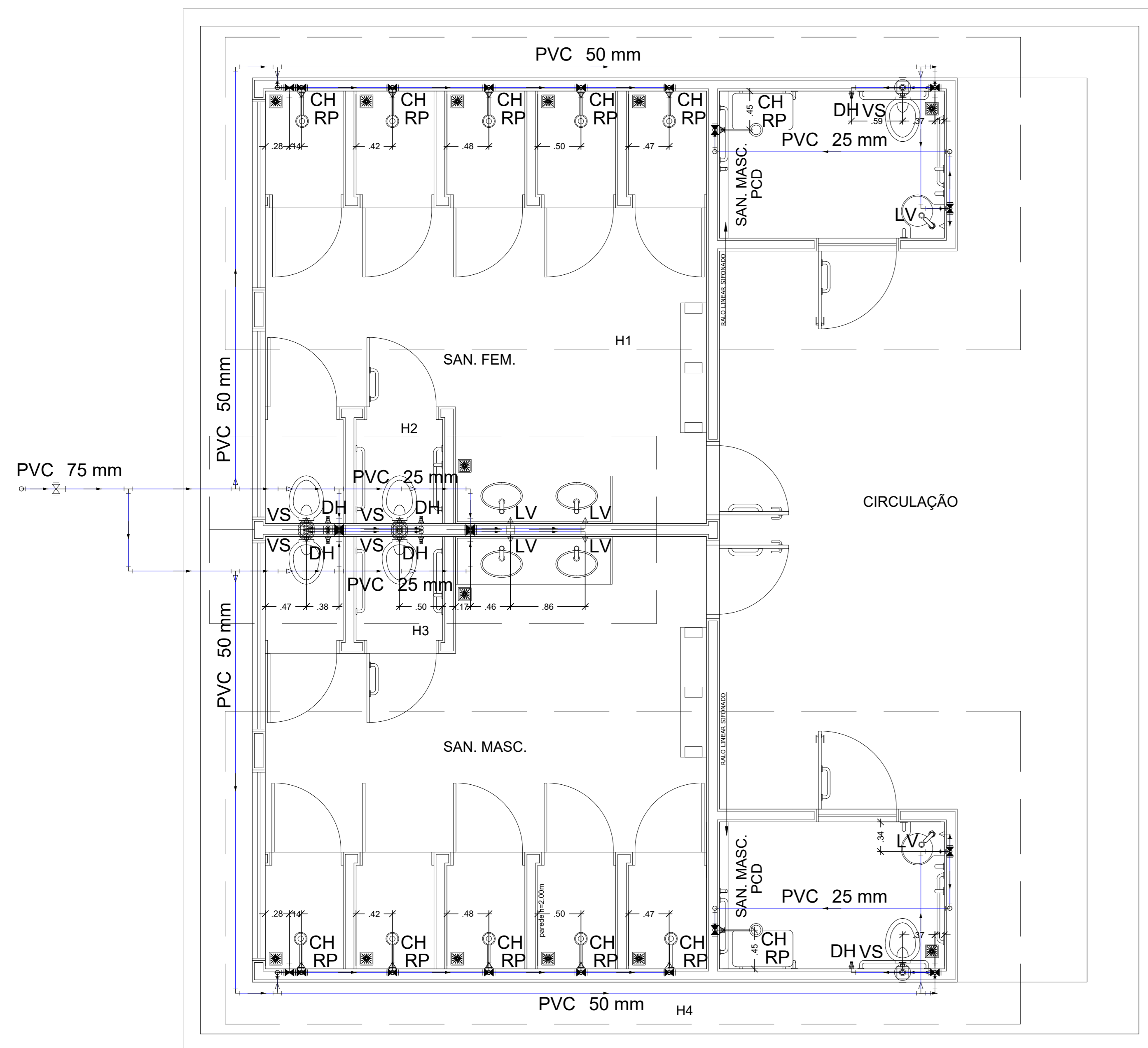
Planta do Terreo - Agua Fria Escala 1:50
